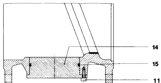
mit Verschlussdeckel / with blind cover
